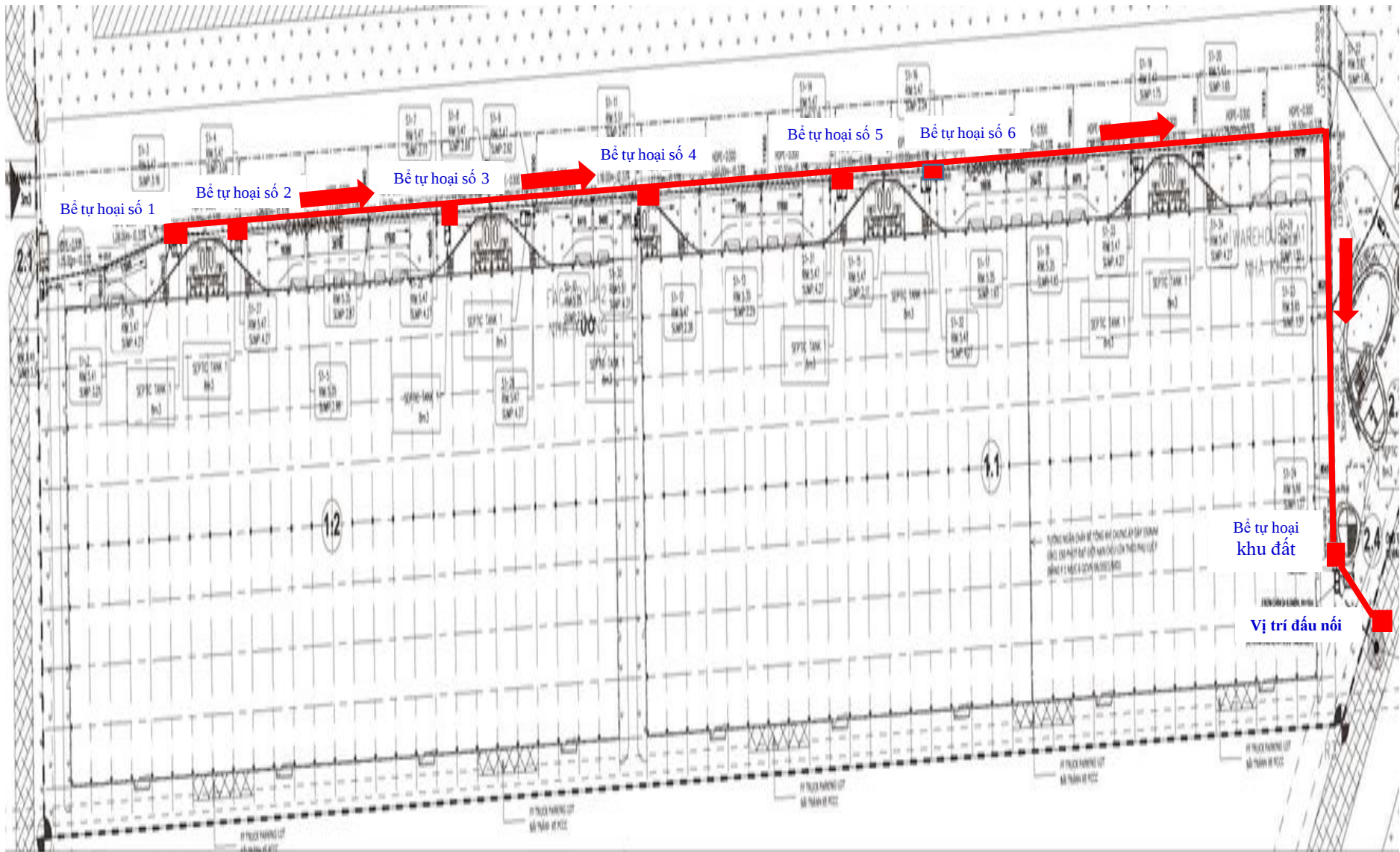
Hình 4. 1. Sơ đồ mạng lưới thu gom và thoát nước thải của dự án
