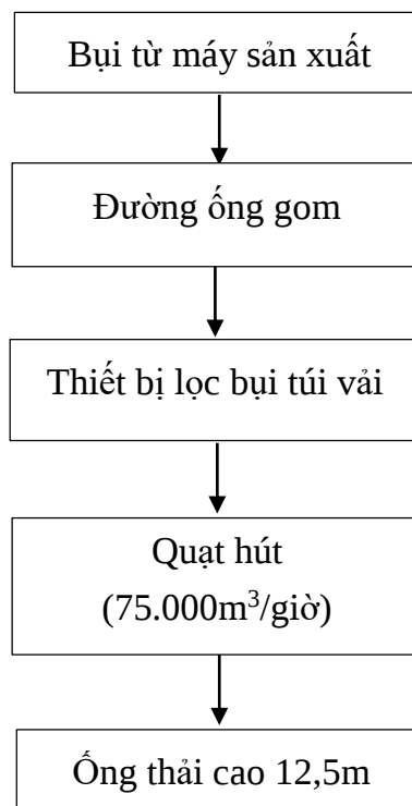
Hình 4. 14. Sơ đồ thu gom xử lý bụi từ máy cắt (cửa nhiều lưỡi)
