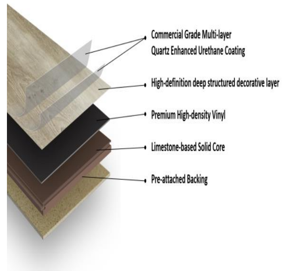
Cấu tạo sàn nhựa WPC
