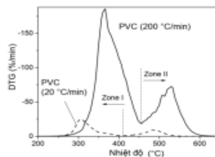
Hình 6. Biểu đồ phân tích nhiệt vi sai (DTG: Derivative thermogravimetric) của PVC trong 2 trường hợp tốc độ gia nhiệt chậm 20^{\circ}C/phút và nhanh 200^{\circ}C/phút thể hiện tốc độ thay đổi trọng lượng theo thời gian hoặc nhiệt độ
