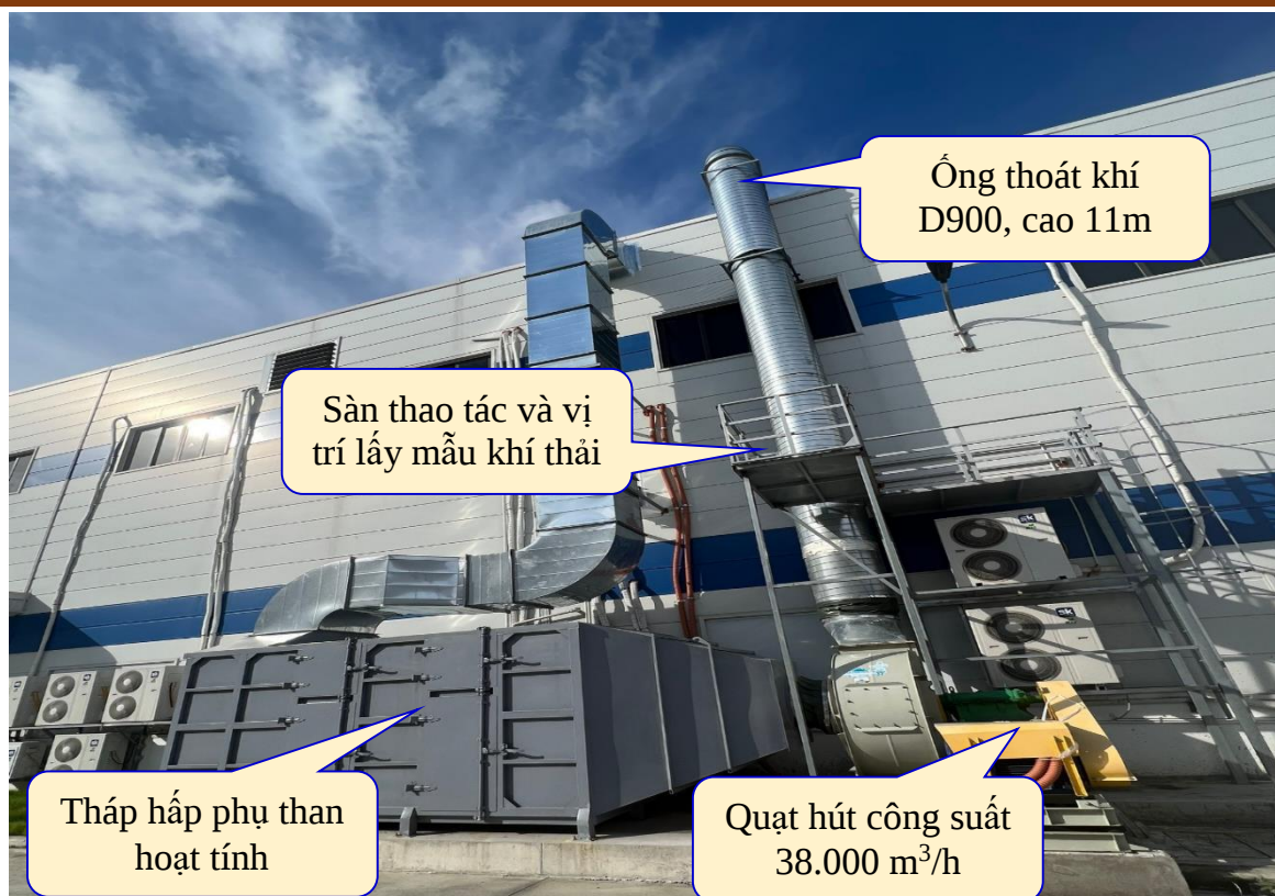
Hình 4. 9. Hình ảnh minh họa hệ thống xử lý khí thải từ chuyền ép đùn
