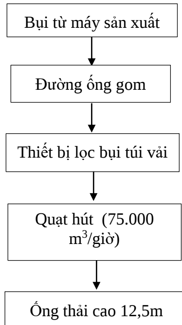
Hình 4. 16. Sơ đồ thu gom xử lý bụi từ chuyền cắt tấm, tạo hèm số 1 và số 2
