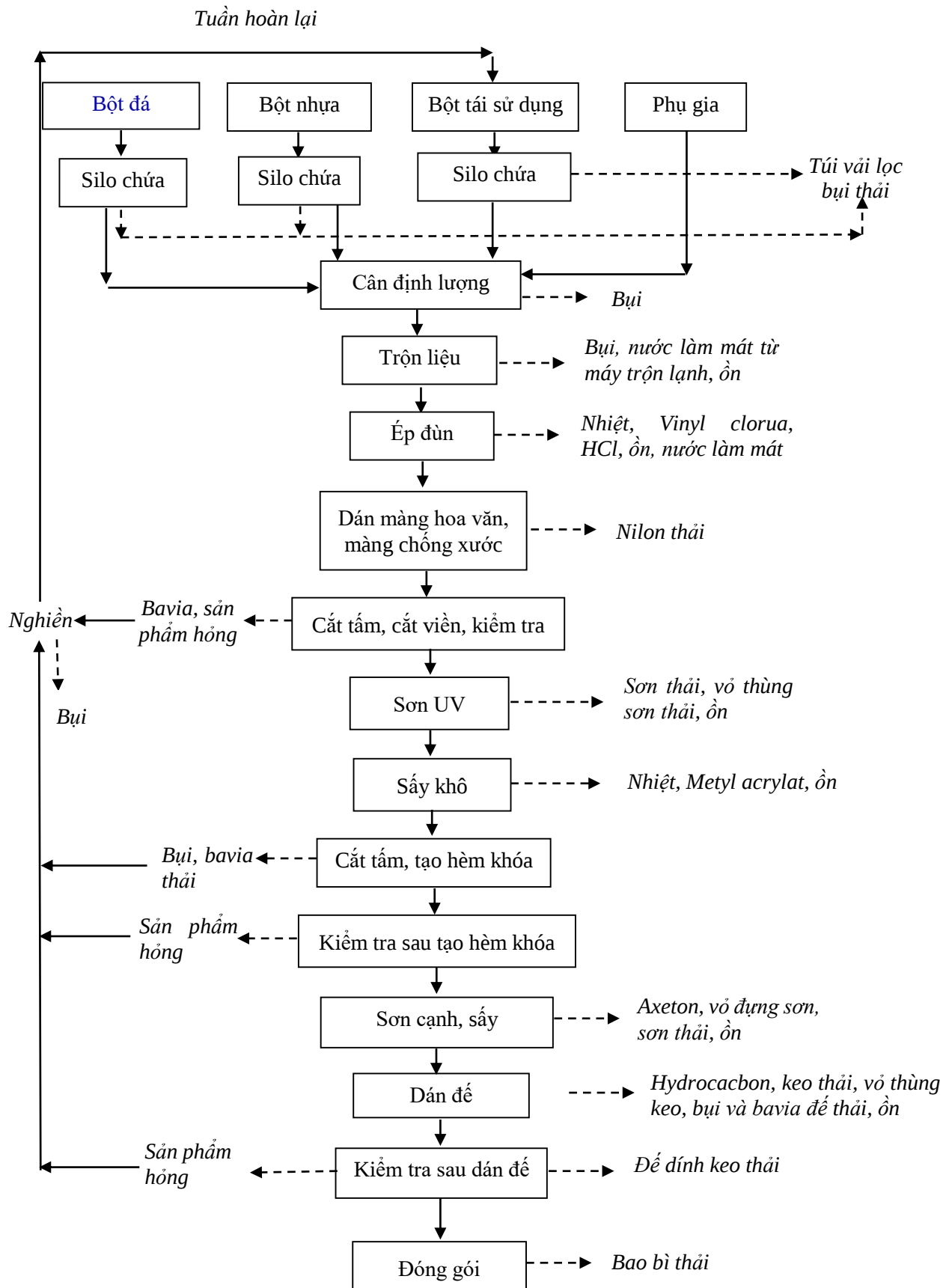
Hình 1. 4. Quy trình sản xuất của dự án
