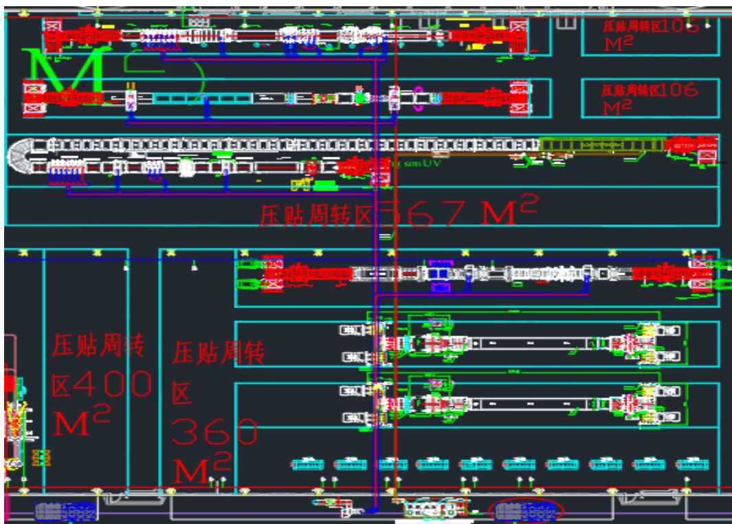
Hình 4. 11. Mặt bằng thu gom và xử lý khí thải từ chuyên sơn và dán đế
