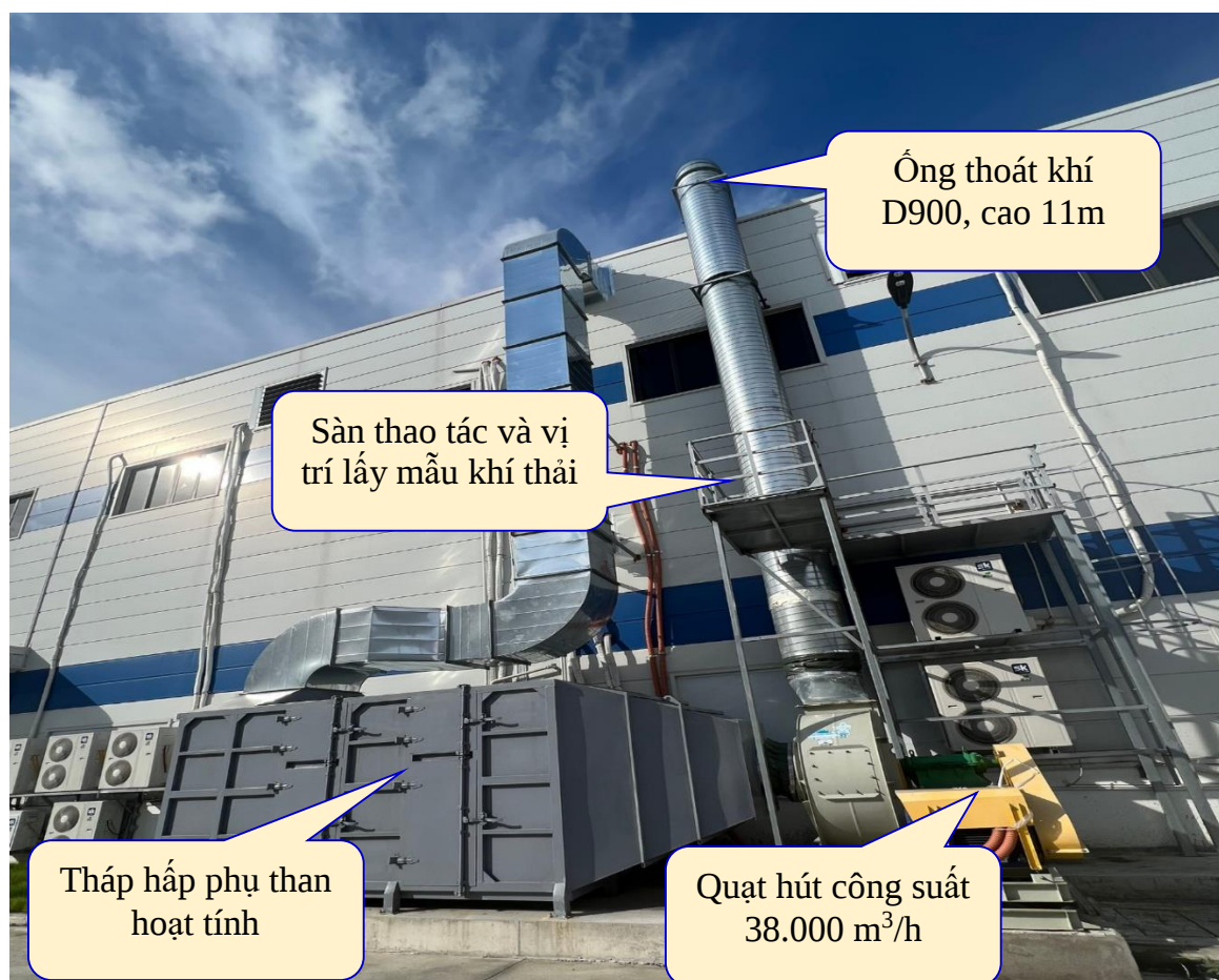
Hình 4. 12. Hình ảnh minh họa hệ thống xử lý khí thải từ chuyên sơn và dán đế
