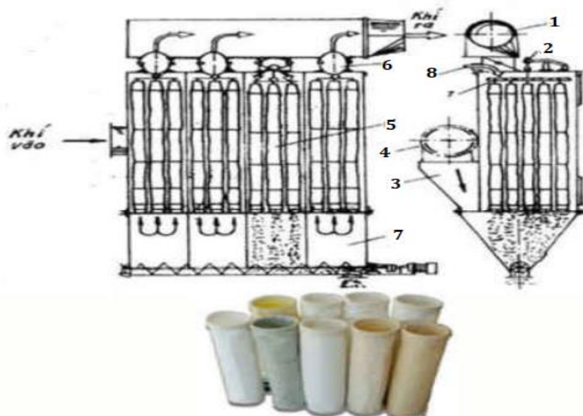
Hình 4. 15. Thiết bị lọc bụi túi vải nhiều đơn nguyên
