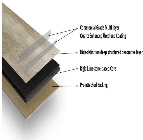
Cấu tạo sàn nhựa SPC
