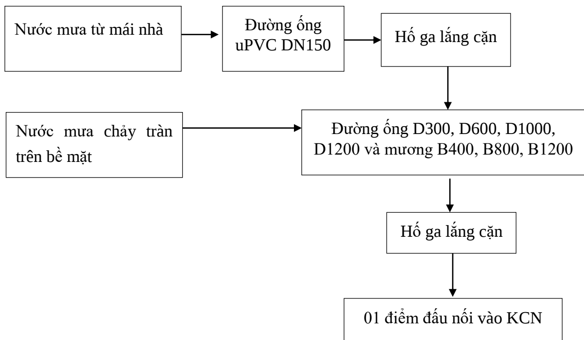
Hình 4. 4. Mạng lưới thu gom nước mưa chảy tràn của dự án
