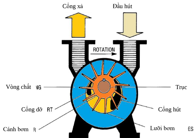
Hình 4. 13. Cấu tạo của bơm chân không vòng nước
