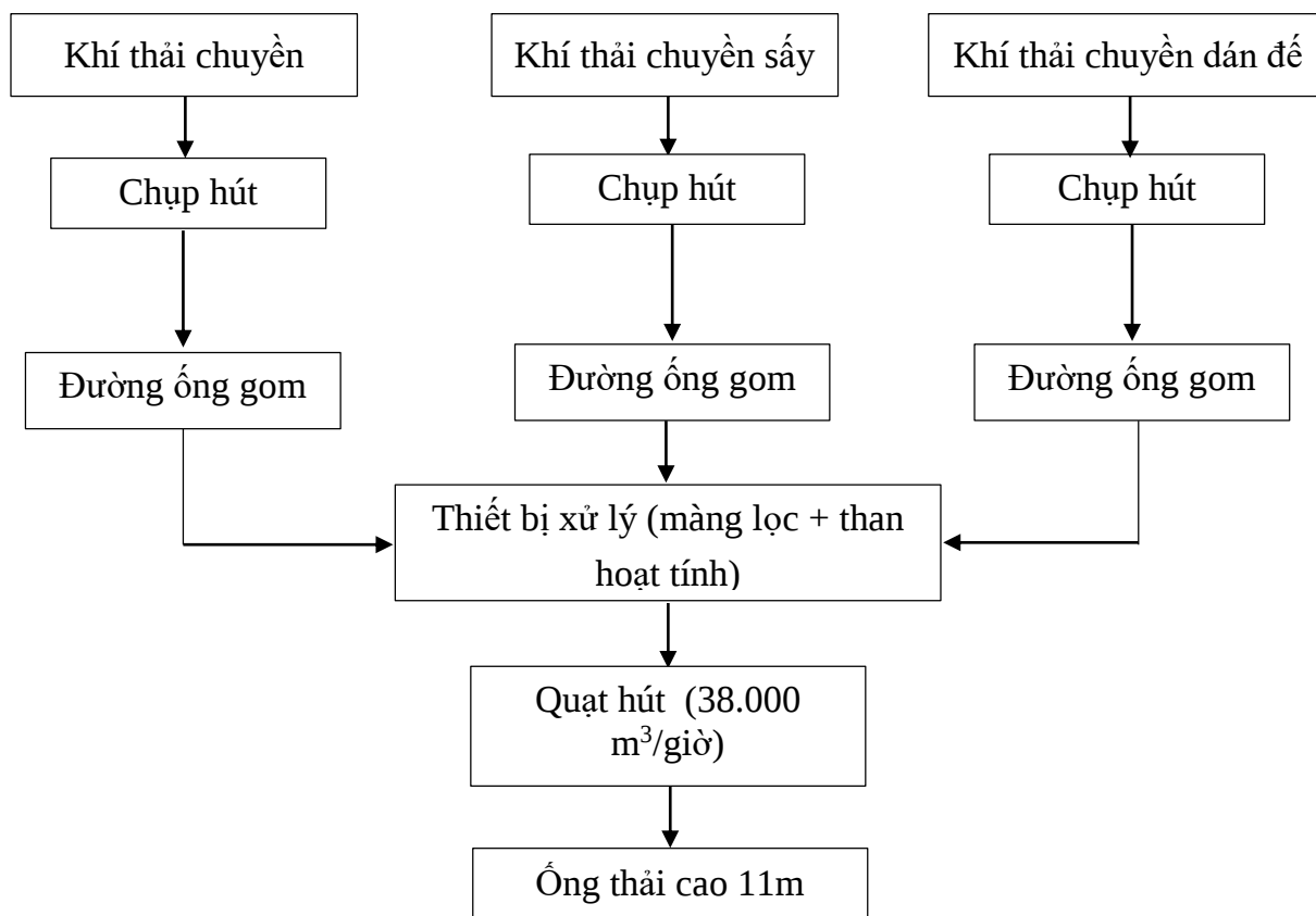
Hình 4. 10. Sơ đồ thu gom xử lý khí thải từ chuyền sơn và dán đế
