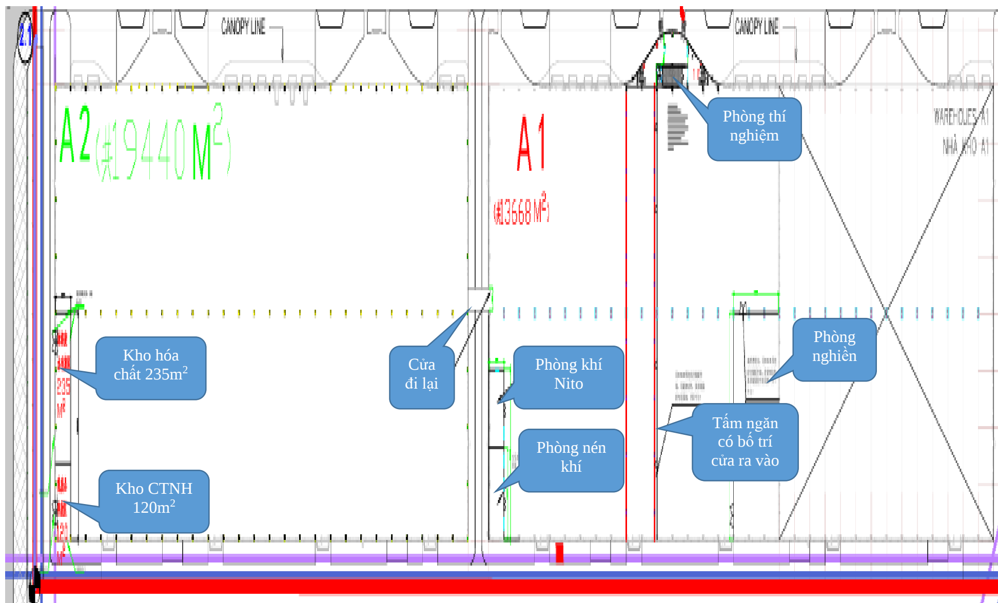
Hình 1. 8. Vị trí thực hiện cải tạo nhà xưởng
