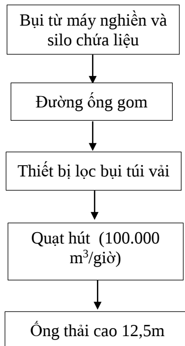
Hình 4. 17. Sơ đồ thu gom xử lý bụi từ máy nghiền
