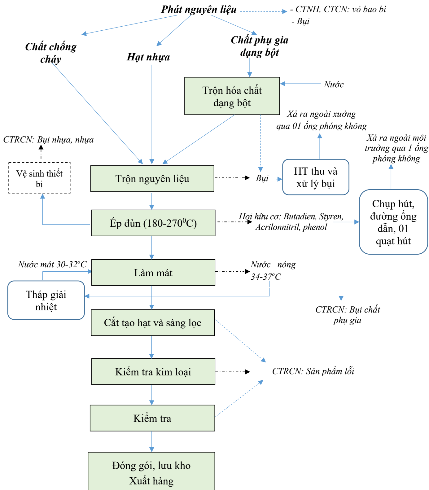
Hình 1.2. Quy trình sản xuất sản phẩm hạt nhựa
